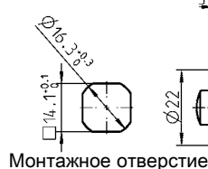
Конструкция А
