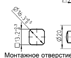
Конструкция В
