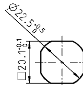
Монтажное отверстие
