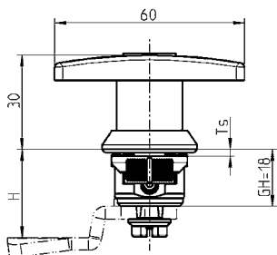
Ригель
