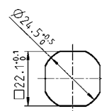
Монтажное отверстие
