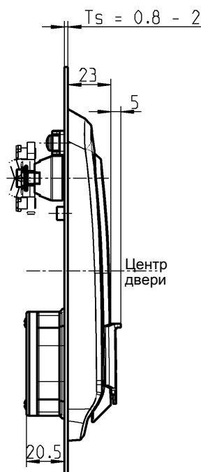
Поворотно-откидная ручка с колпачком и переходником для ригеля
