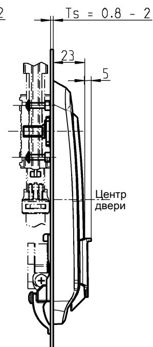
Поворотно-откидная ручка с крючком для замка с тягой
