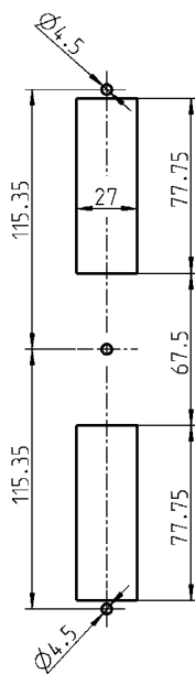
Монтажное отверстие
